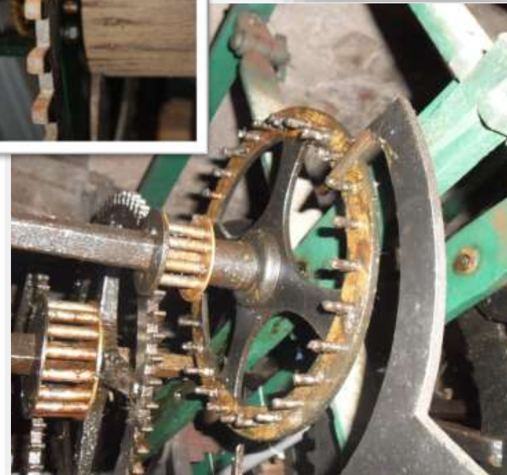
Torenuurwerk Idaerd 1573, één van de oudsten uit Friesland
