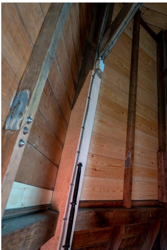
Aangelaste hoekkeper.
